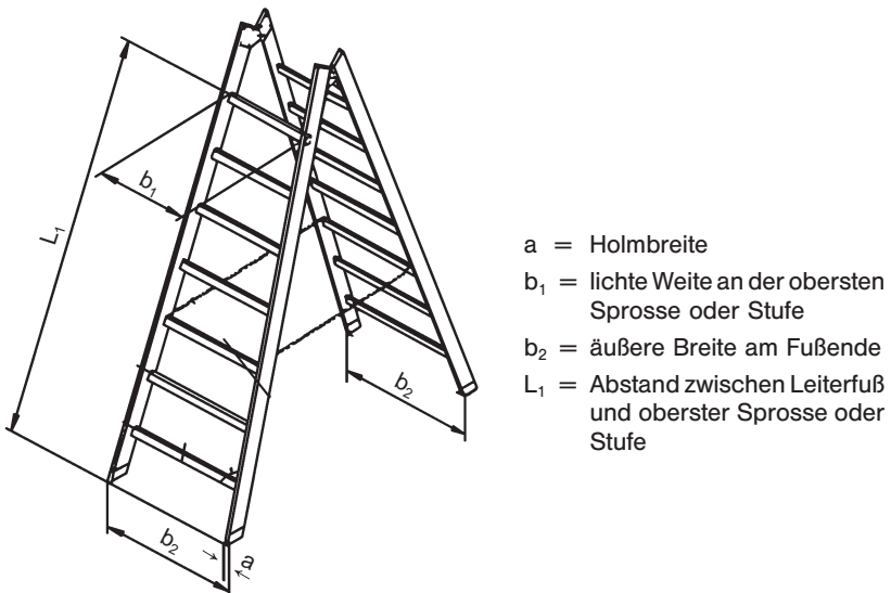
Bild 3: Stehleiter mit sich verjüngenden Leiterschenkeln (Konizität)
