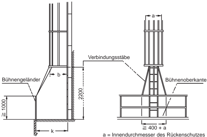
Bild 6: Steigleiter mit verlängertem Rückenschutz durch Verbindungsstäbe
